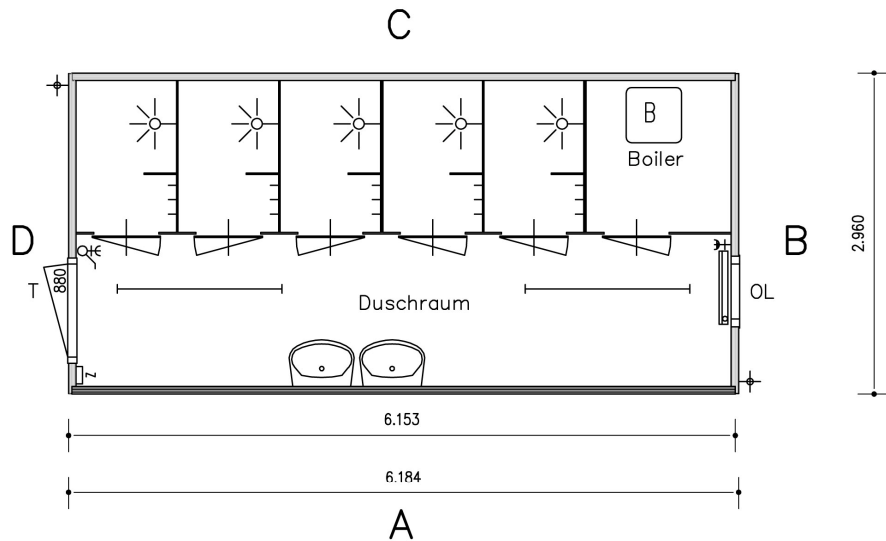
Grundriss
