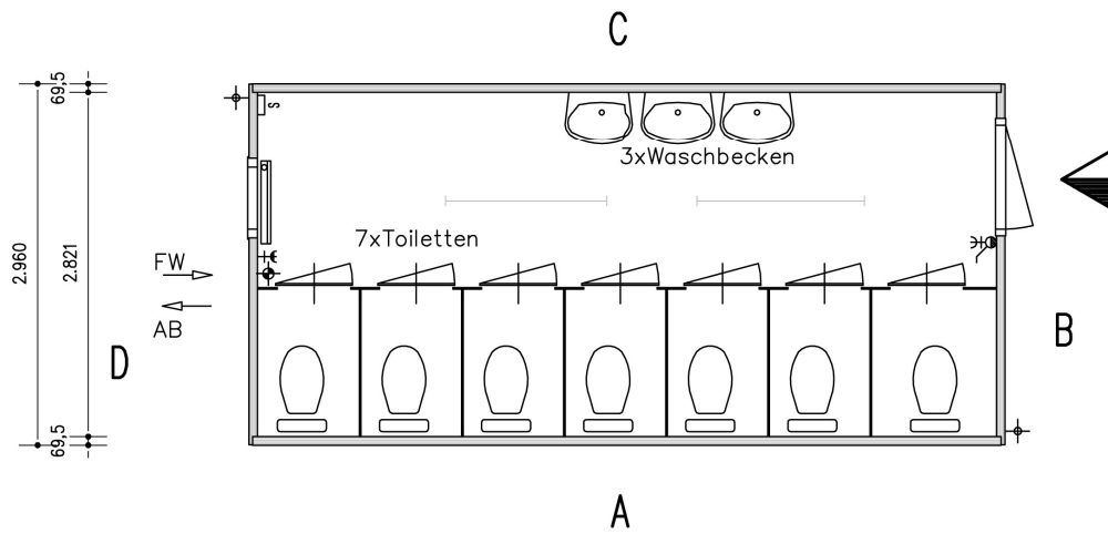
Grundriss
