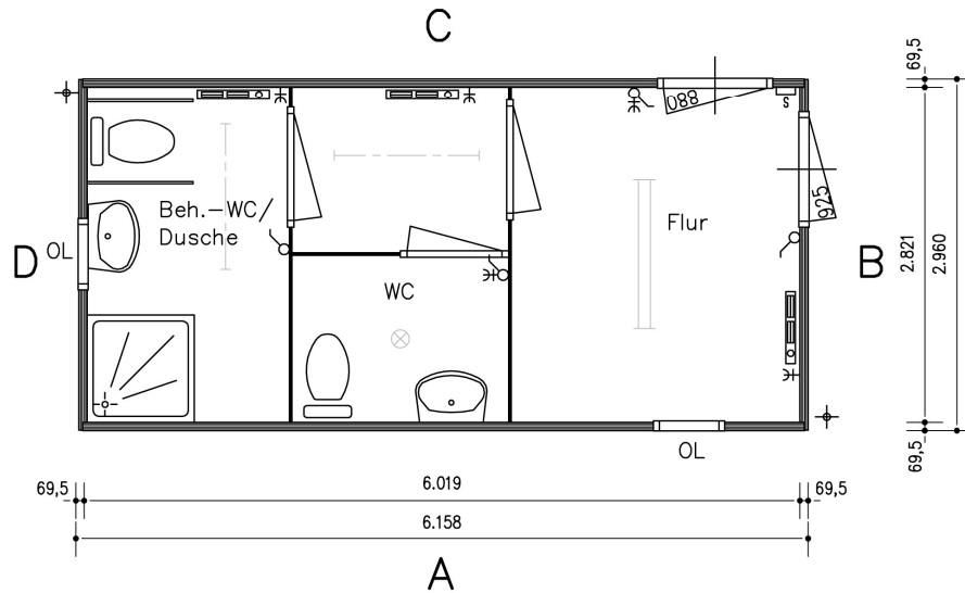
Grundriss
