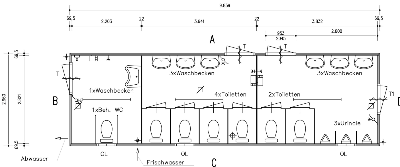
Grundriss
